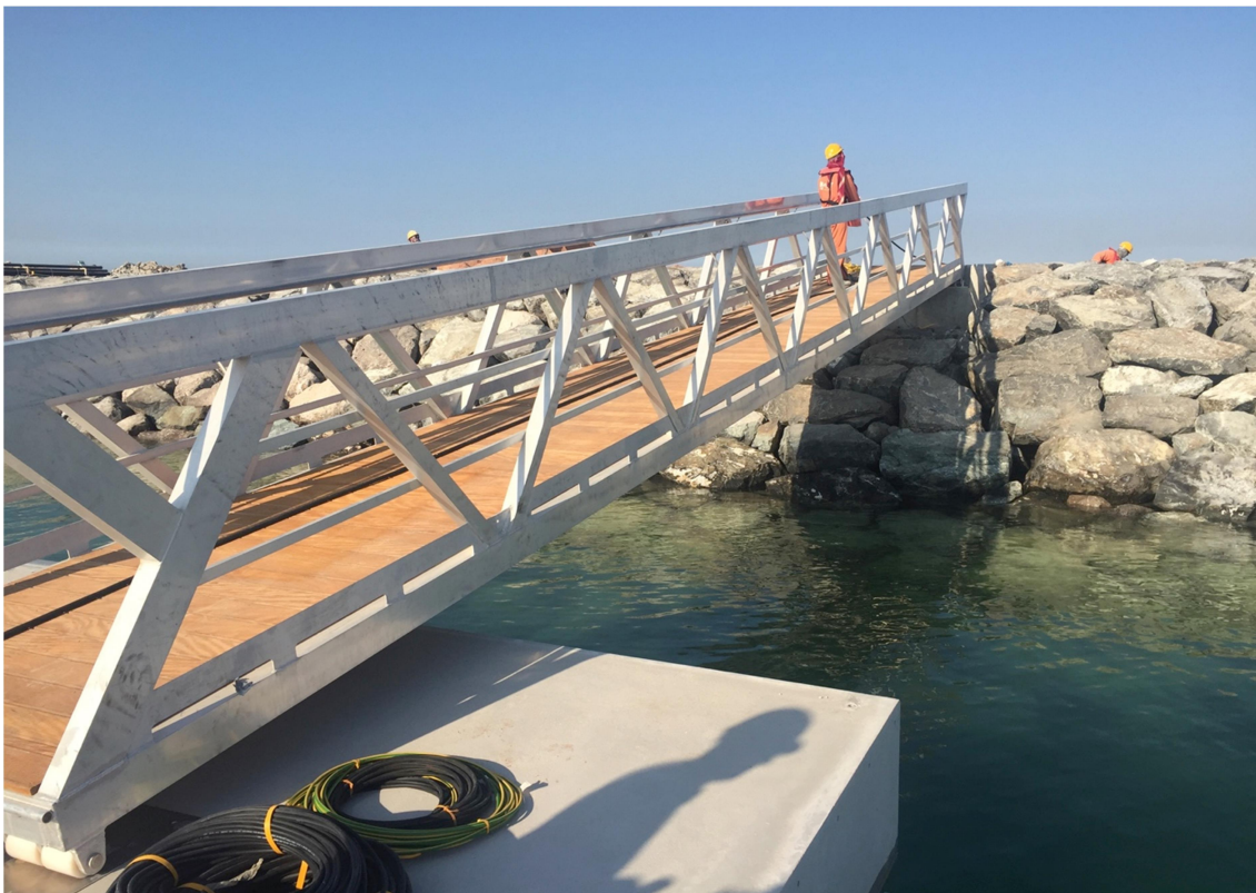
Fig 15. Aluminium access gangway
